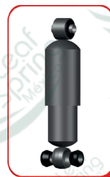
Superior: Anillo / Buje / Camisa Inferior: Anillo / Buje Trapezoidal Abreviatura: ABC / ABT
